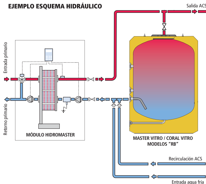
EJEMPLO ESQUEMA HIDRÁULICO
