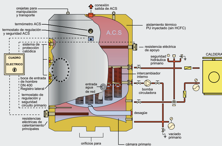
MODELOS MVV-1500...4000/ESSB. INSTALACIÓN "CALDERA / ELÉCTRICO" calentamiento combinado
