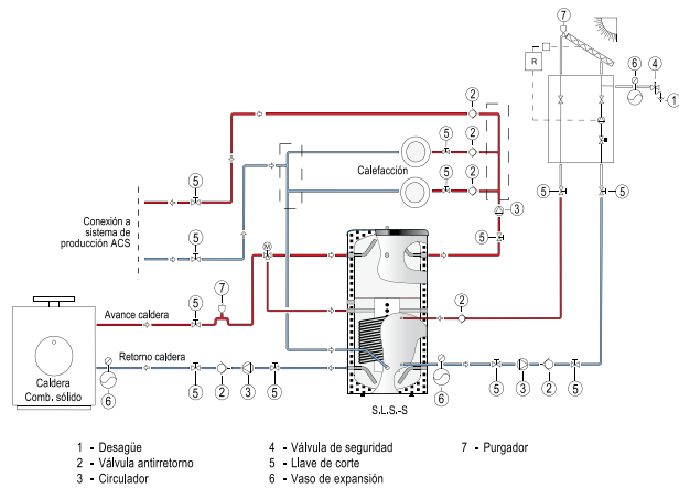
Centro energético de acumulación (LW) Conexión a sistema de producción mediante intercambiador de placas o productor/acumulador de ACS.
