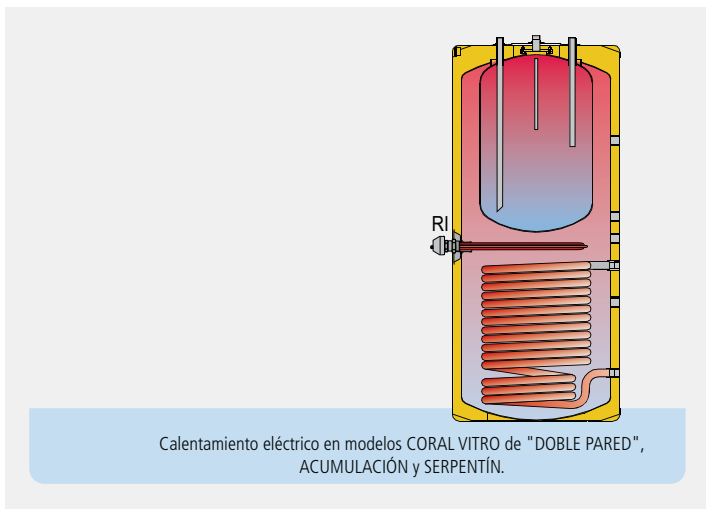
RESISTENCIAS "RI": Resistencias roscadas de inmersión, para circuito primario de calentamiento, en modelos CORAL VITRO de "DOBLE PARED"
