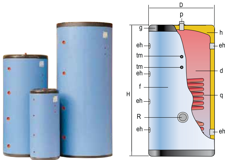
d - Depósito de inercia f - Forro externo g - Cubierta h - Aislamiento térmico q - Serpentin intercambiador
