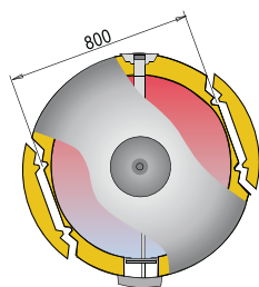
Detailansicht der abnehmbaren Dämmschicht bei 800 und 1000 Liter Speichern für Montageöffnungen ab 800 mm
